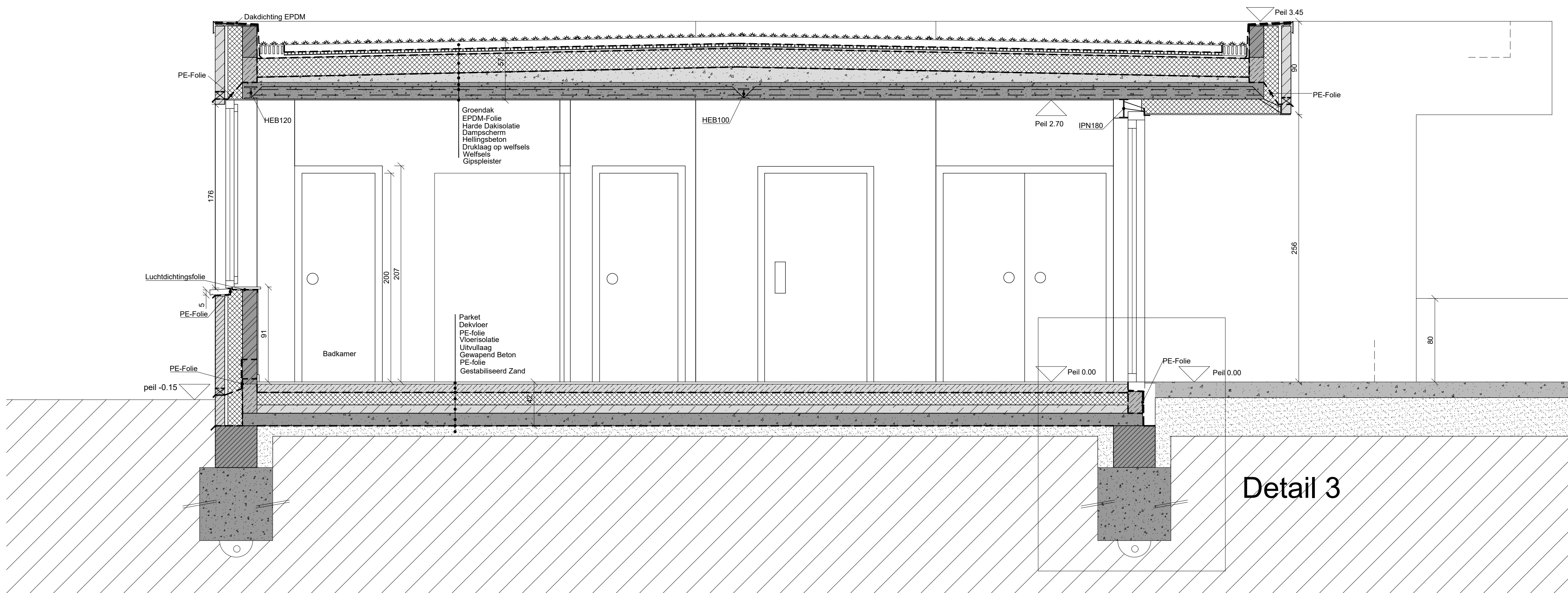
Doorsnede BB' 1/25
