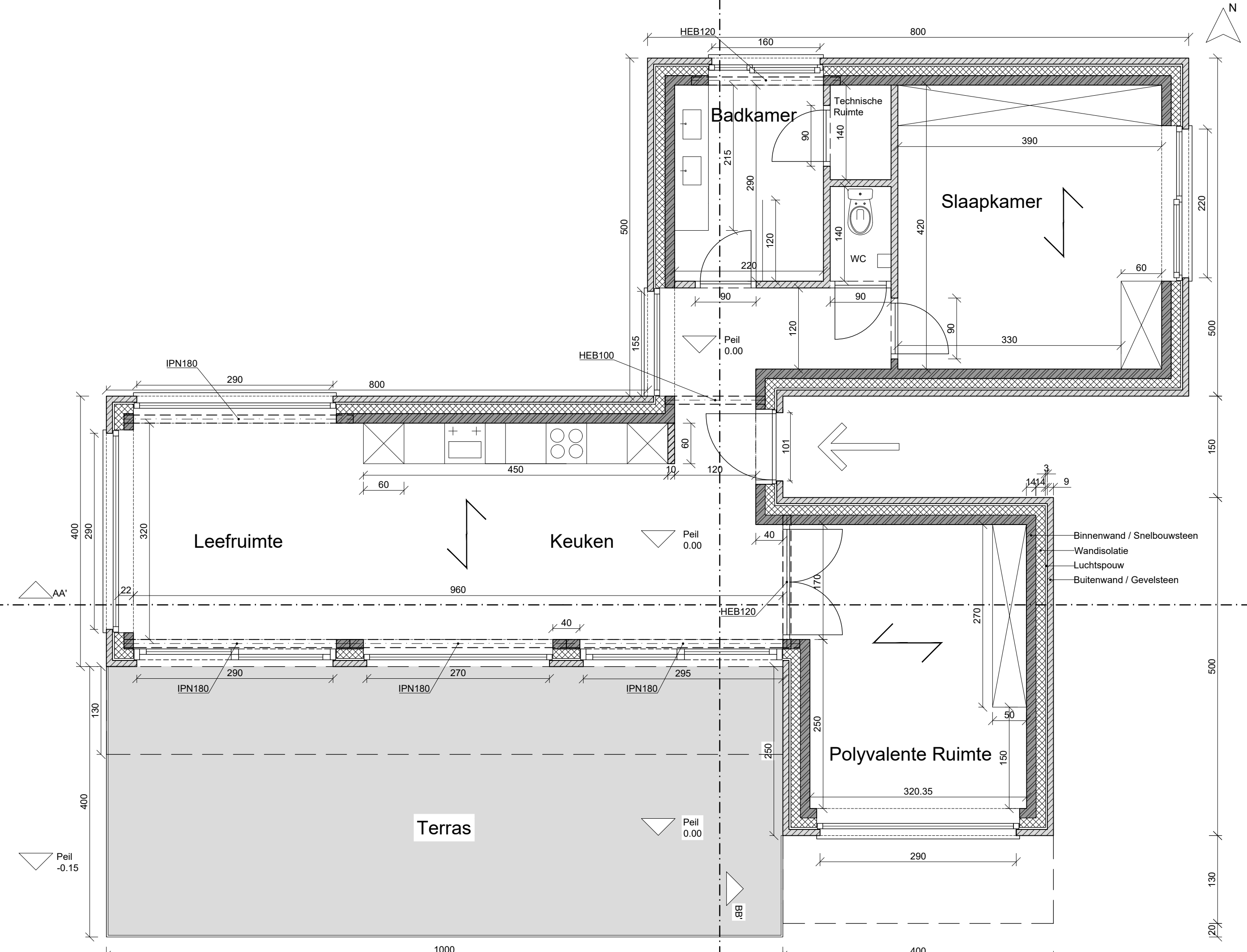
Grondplan 1/50
