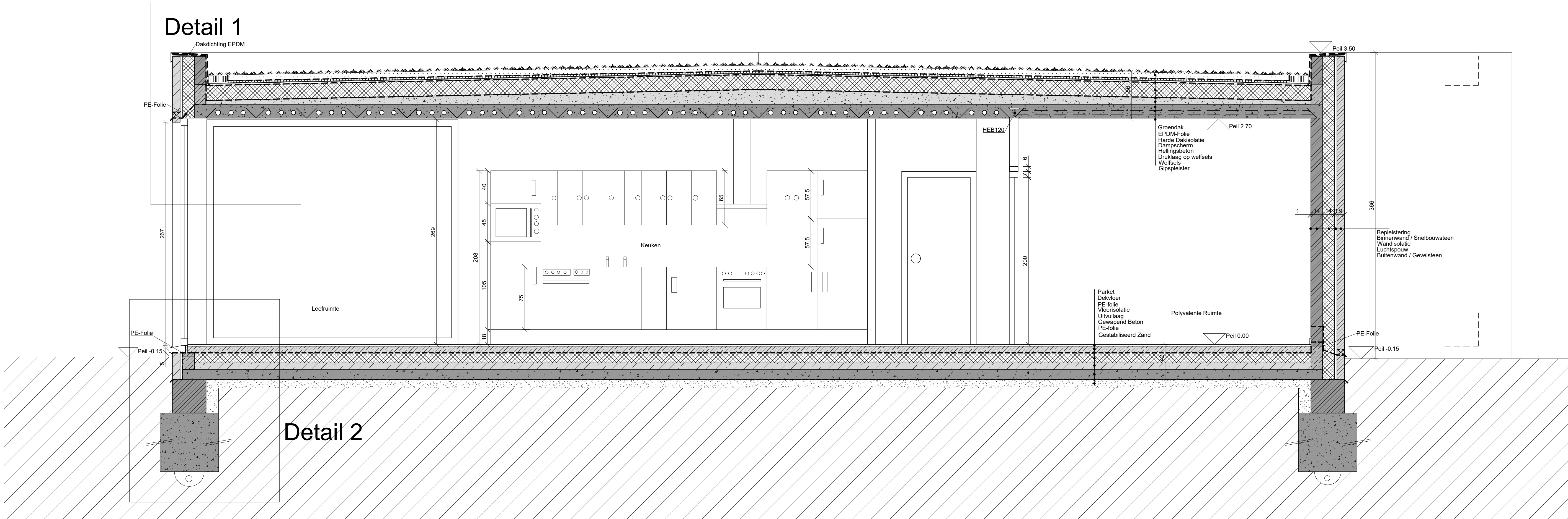
Doorsnede BB' 1/25
