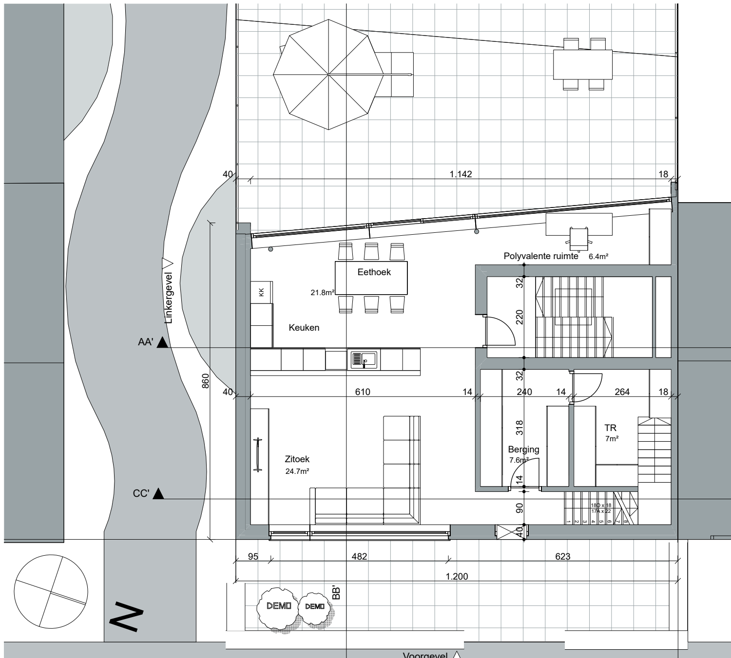
Grondplan Eerste Verdiep
