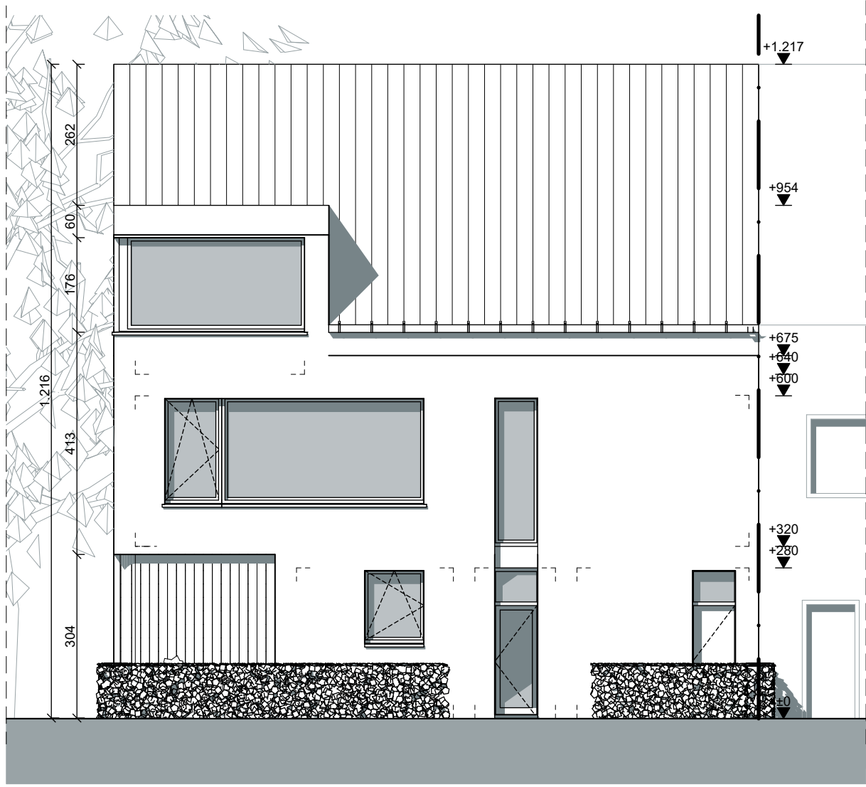
Voorgevel / Noordoostgevel
