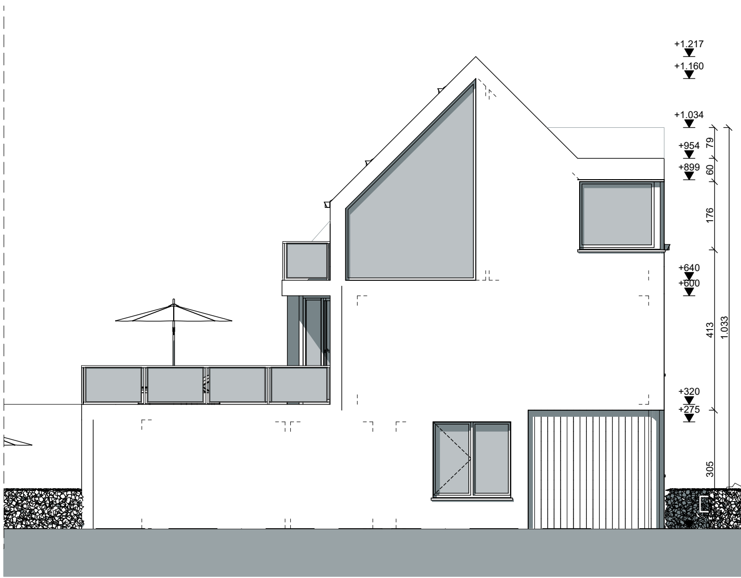
Zijgevel / Zuidoostgevel
