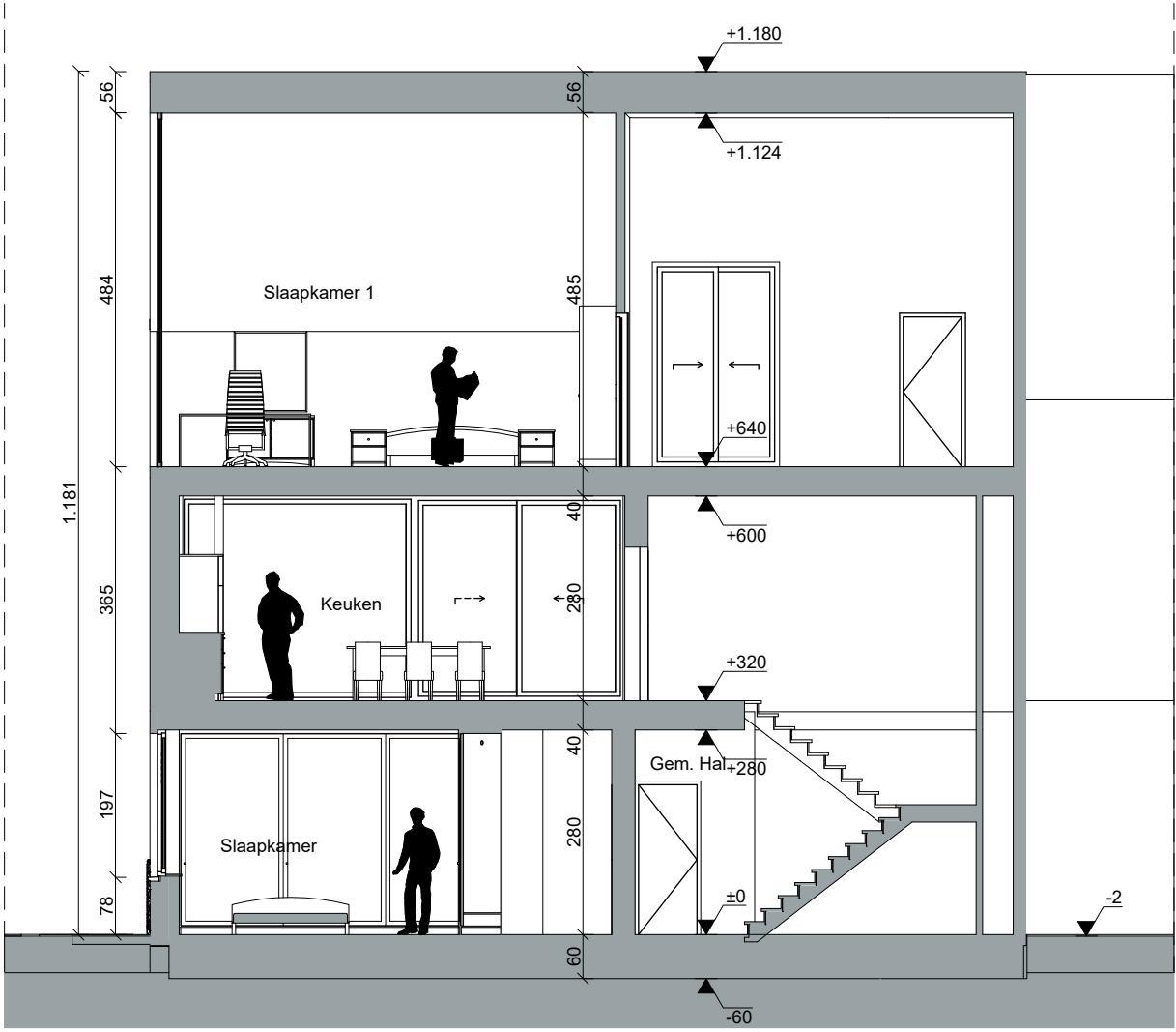
Sneede AA'
