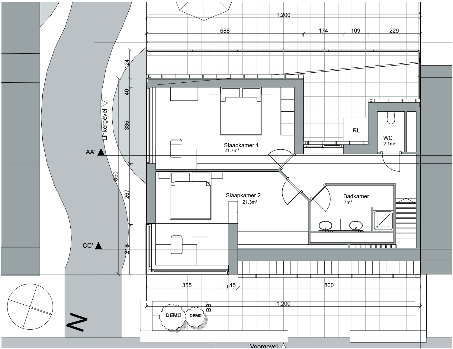
Grondplan Tweede Verdiep
