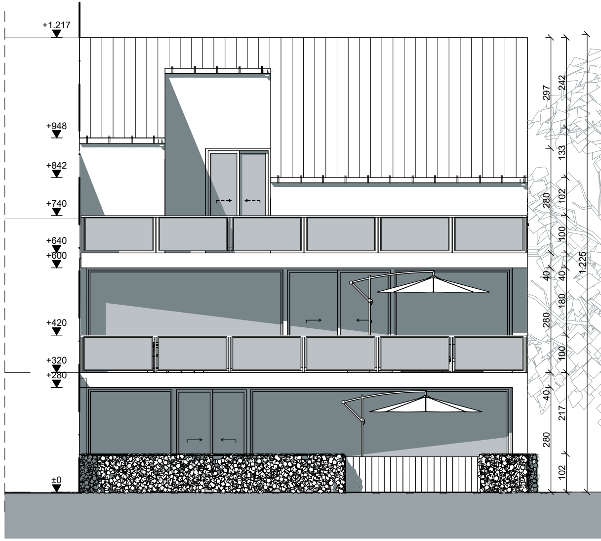
Achtergevel / Zuidwestgevel
