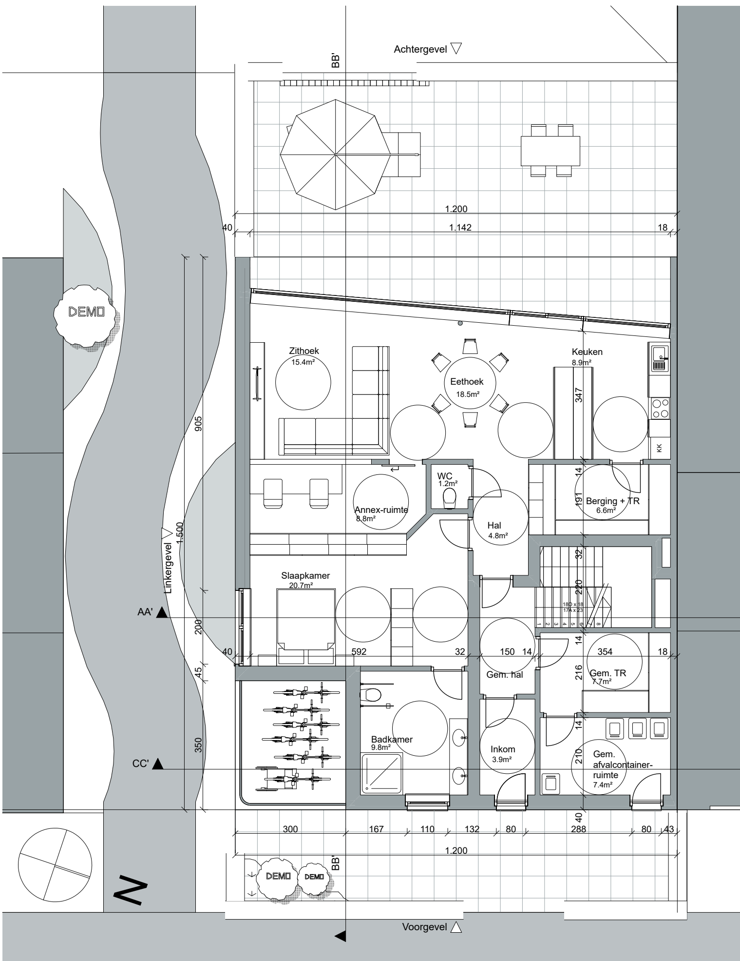
Grondplan Gelijkvloers
