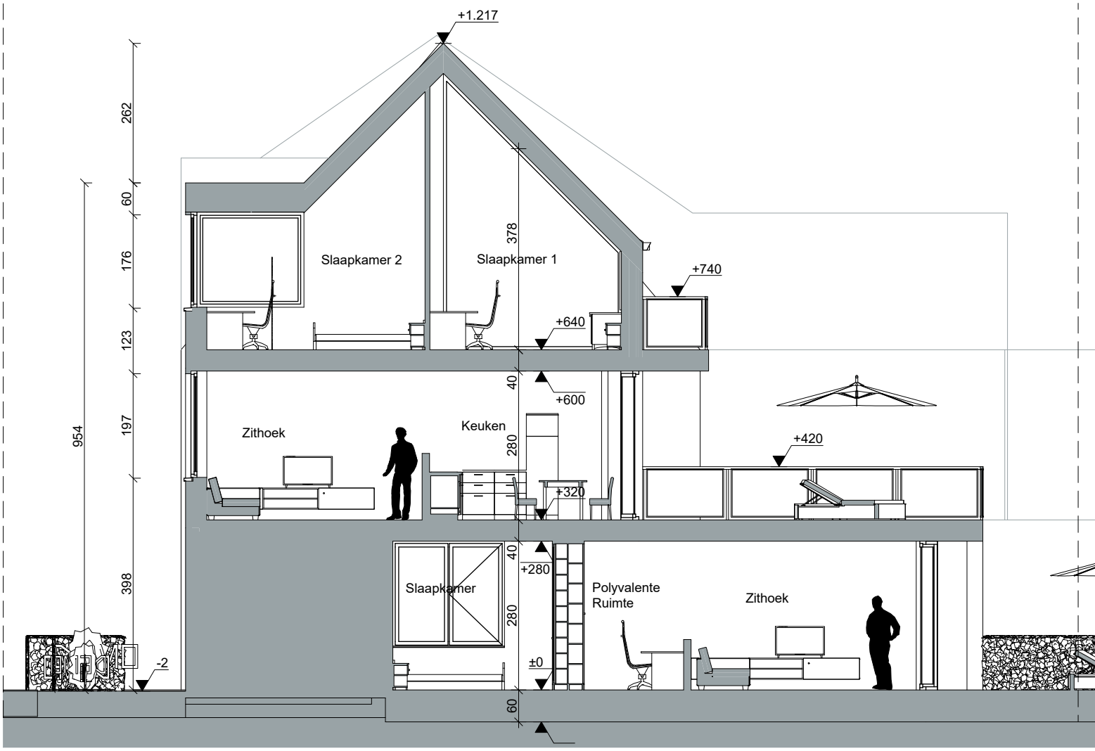
Sneede BB'
