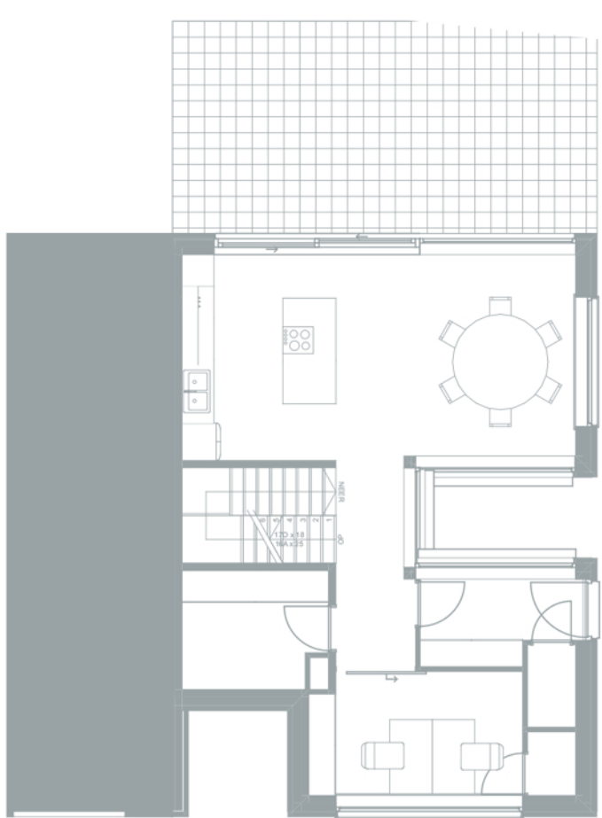
Gelijkvloers Archicad
