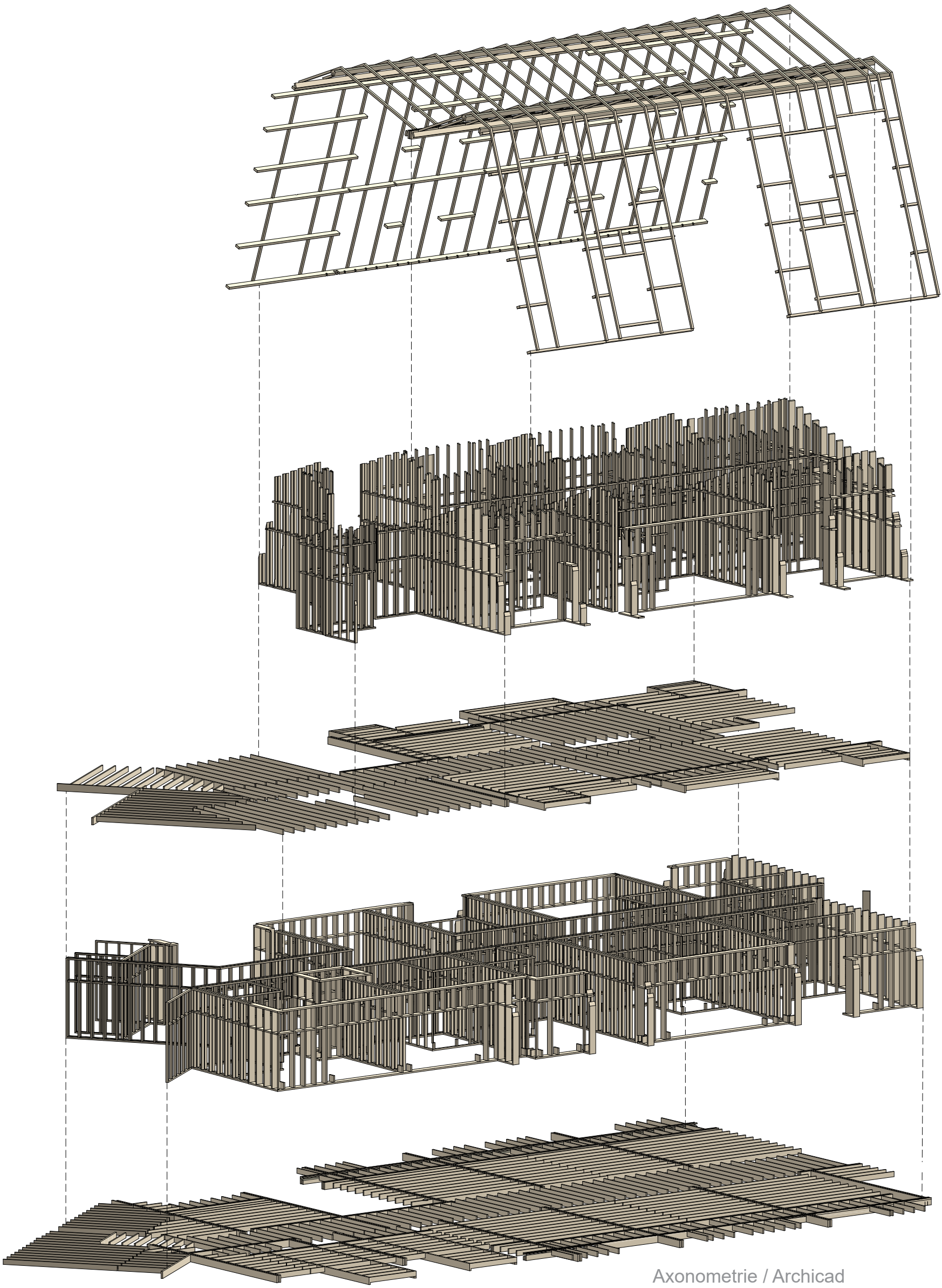
Axonometrie / Archicad
